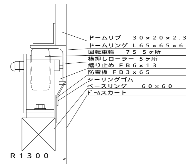
A - A 断面図 1 / 2
